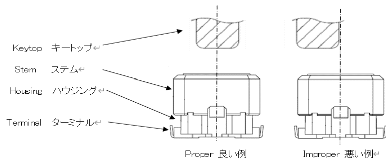
Fig 2: Keytop and Stem relationship 図 2: キートップとステムの関係
